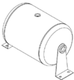
SERBATOIO STL: staffe fornite separatamente
